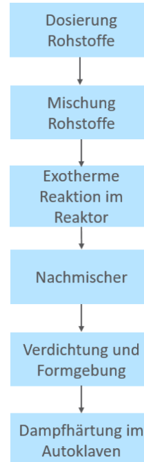
Abbildung 1: Produktherstellung
